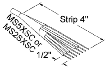
Figure 11 – MS5XSC/MS2SXSC Wiring
